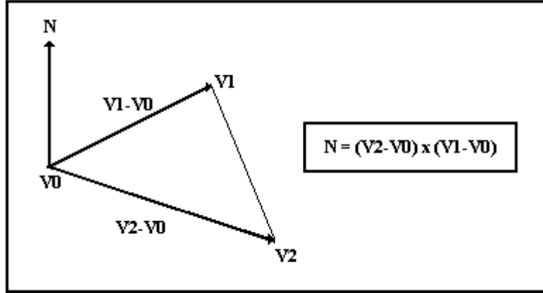
Şekil 1.4. Yüzey normalinin hesaplanması
