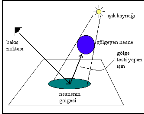
Şekil 1.16. Işın izleme ile gölge testi
