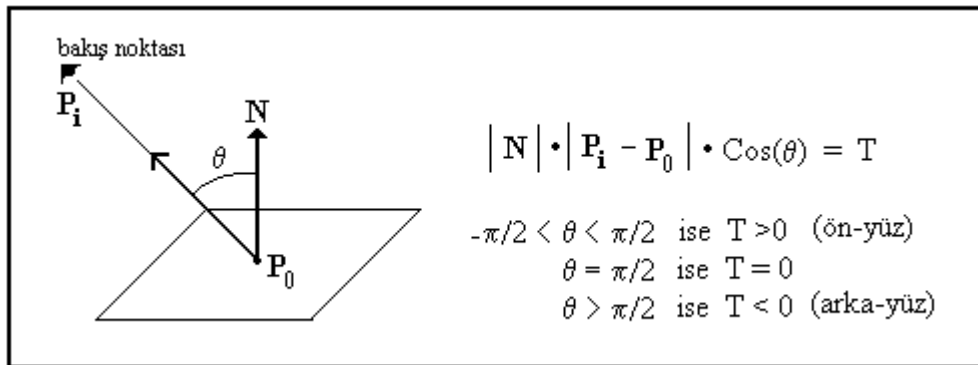
Şekil 1.33. Skaler çarpımla arka-yüz kaldırma
