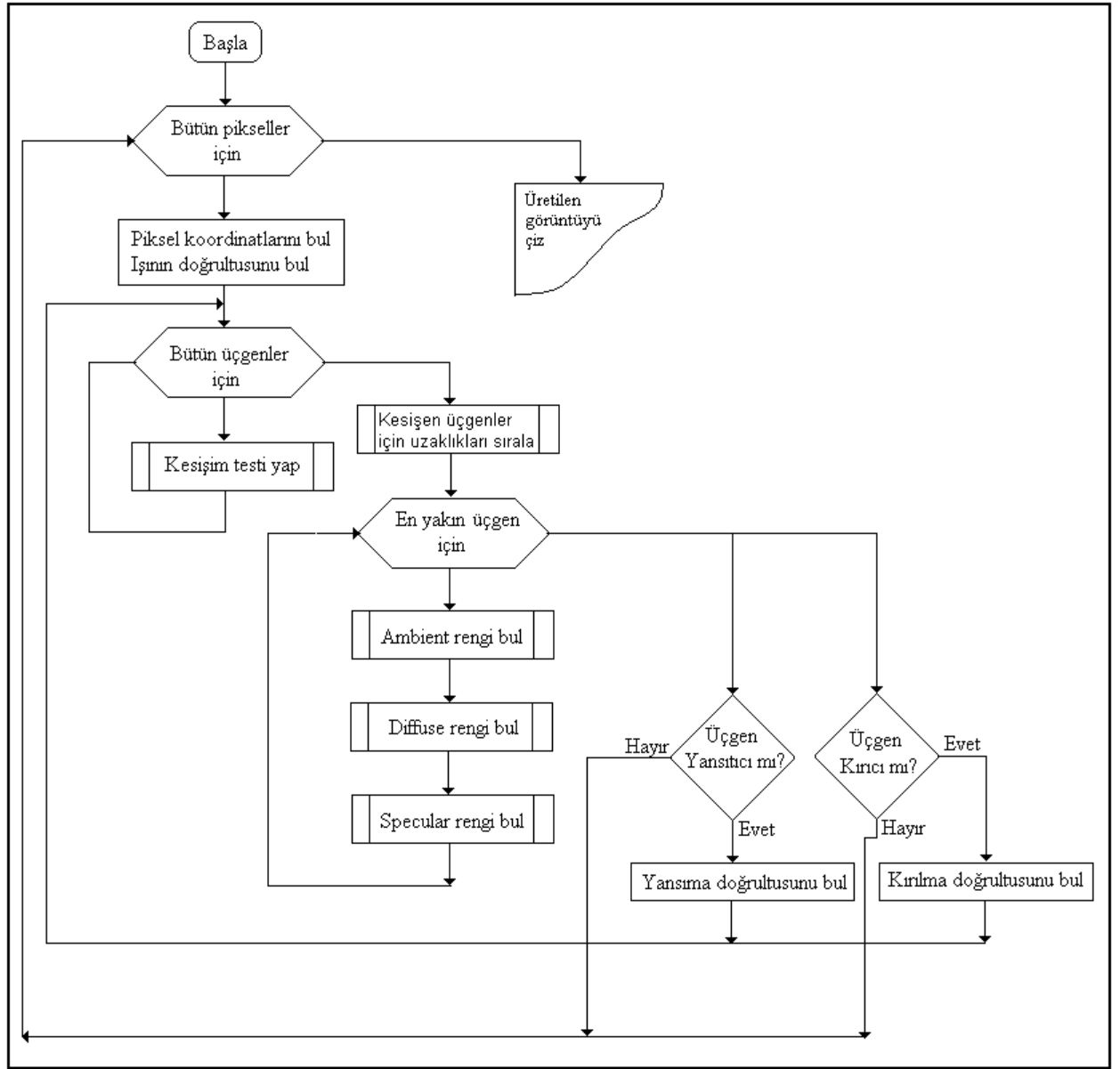
Şekil 2.11. Özyinelemeli ışın izleme programının akış diyagramı
