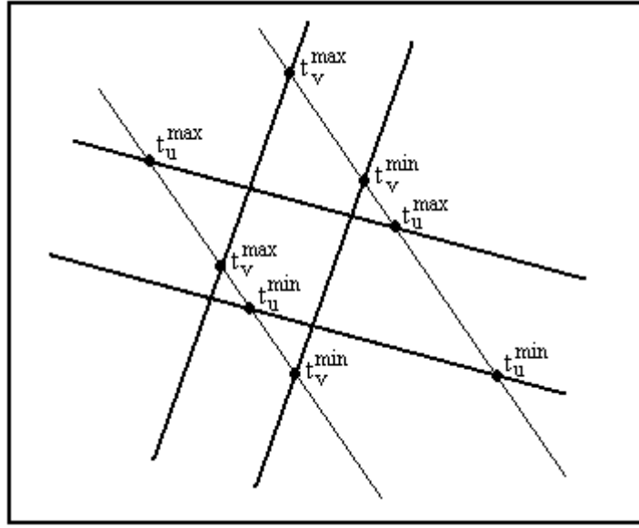
Şekil 1.35 u-v eksenine için min. ve max. t değerleri
