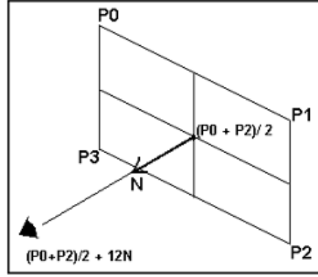
Şekil 2.22. Etkileşimli ışın izleme
