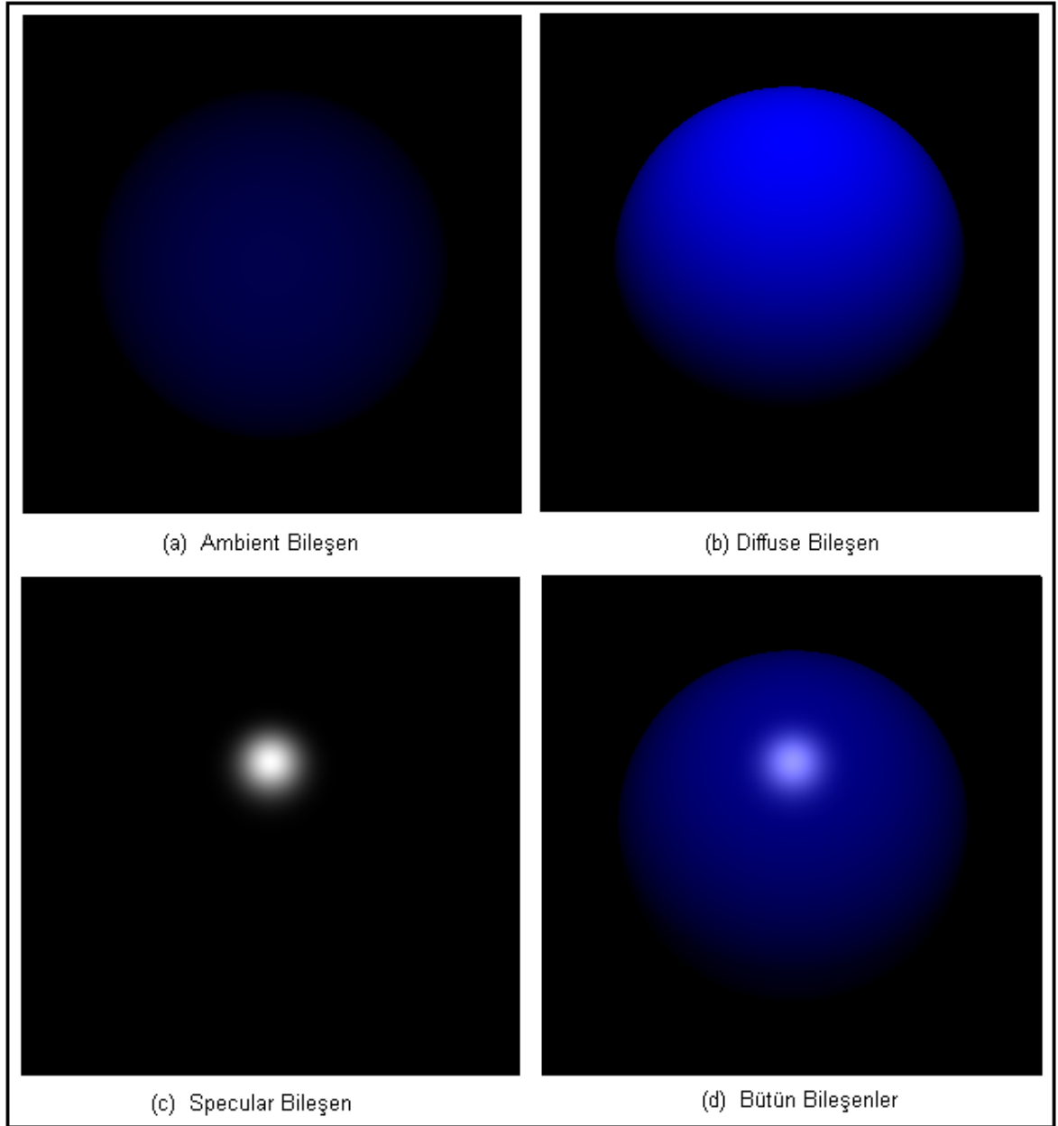
Şekil 1.25. Aydınlatma modelinin bileşenleri
