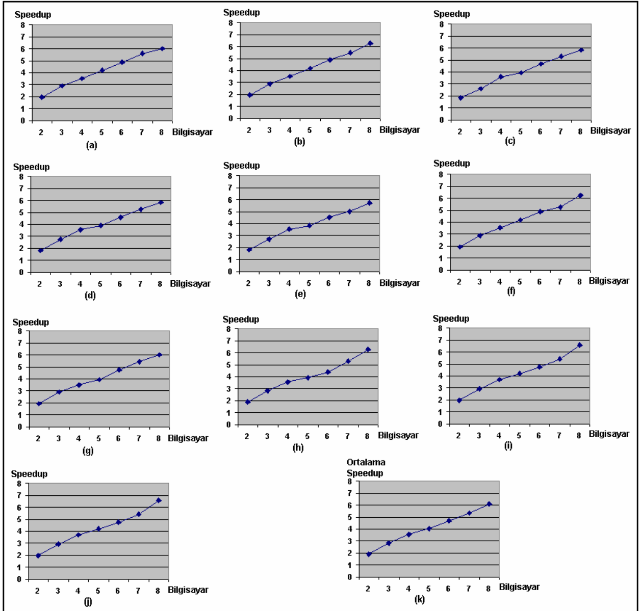
Şekil 3.1. Paralel etkileşimli ışın izleme ile üretilen görüntüler için speedup eğrileri
