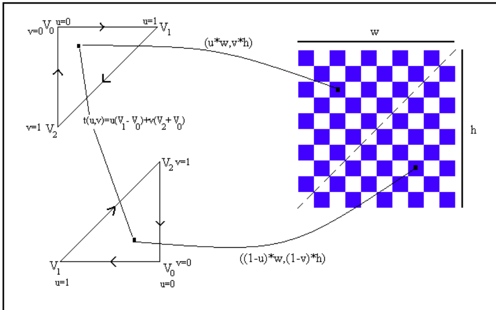
Şekil 1.26. Barisentrik koordinatlarla doku kaplama
