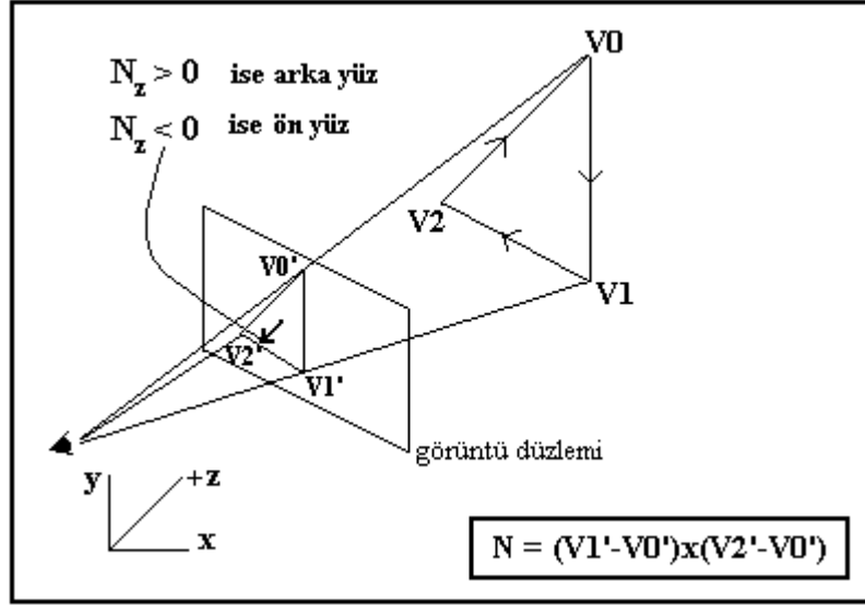
Şekil 1.32. Vektörel çarpımla arka-yüz kaldırma
