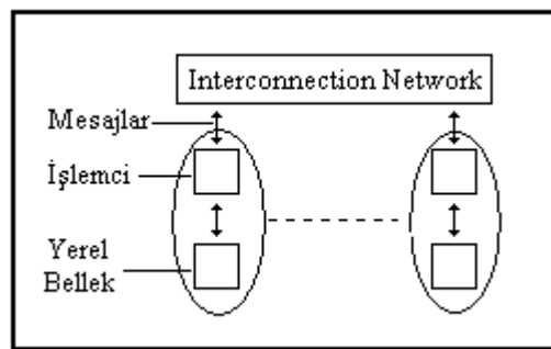
Şekil 1.37. Mesaj-geçmeli çoklu-bilgisayar sistemi
