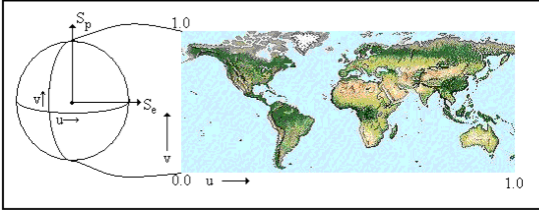
Şekil 1.27. Küre üzerine doku kaplama.
