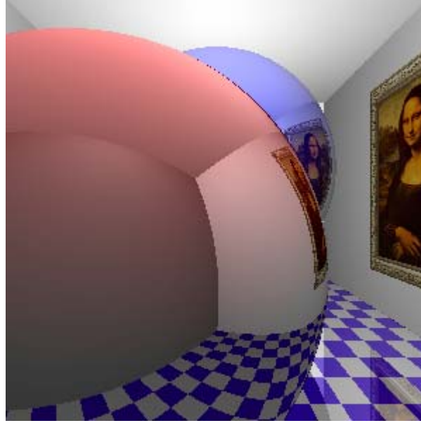
Şekil 2.6. Yansıma, derinlik=1
