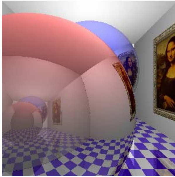
Şekil 2.8. Yansıma, derinlik=3
