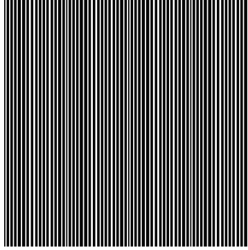
Şekil 2.16. Bump dokusu
