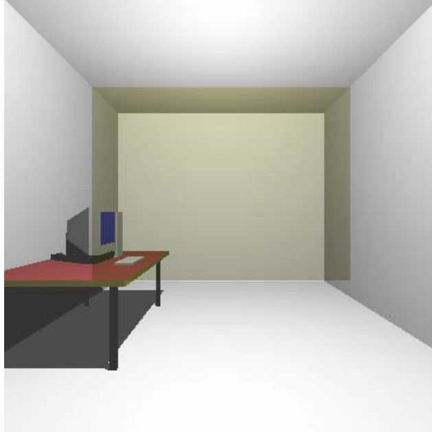
Şekil 2.10. Saydam yüzey
