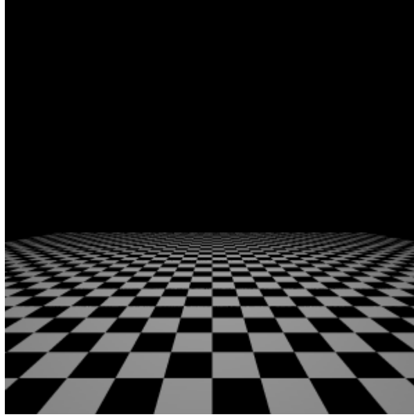
Şekil 1.31. Antialiasing
