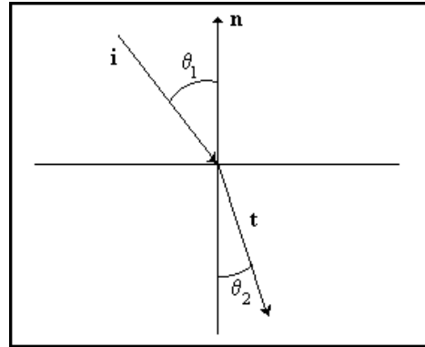
Şekil 1.20. Snell kanununa göre ışının kırılması
