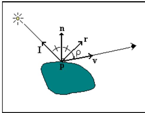
Şekil 1.22. Specular bileşen
