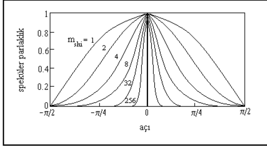
Şekil 1.23. Parlaklık parametresinin değışimi
