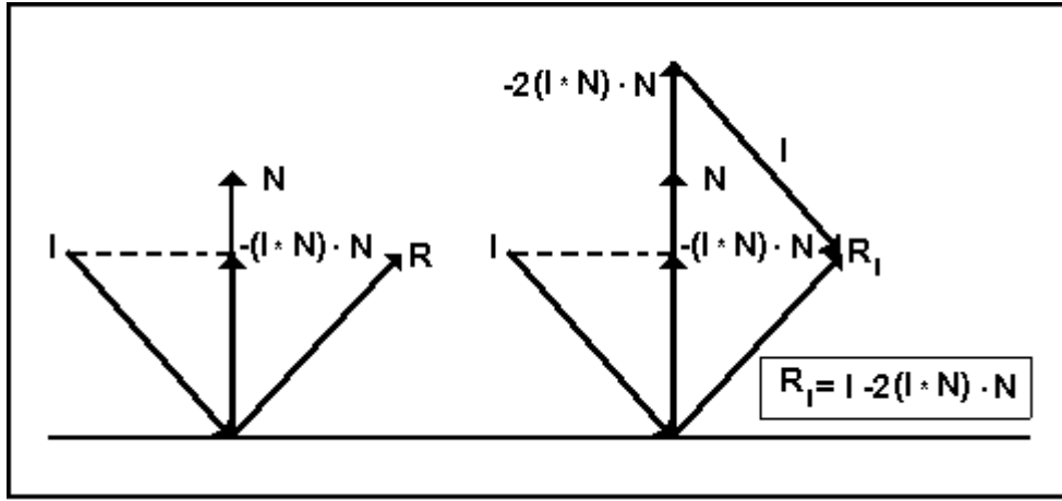
Şekil 1.17. Yansıyan ışının doğrultusu \mathbf{R}_1 ‘nın hesaplanması
