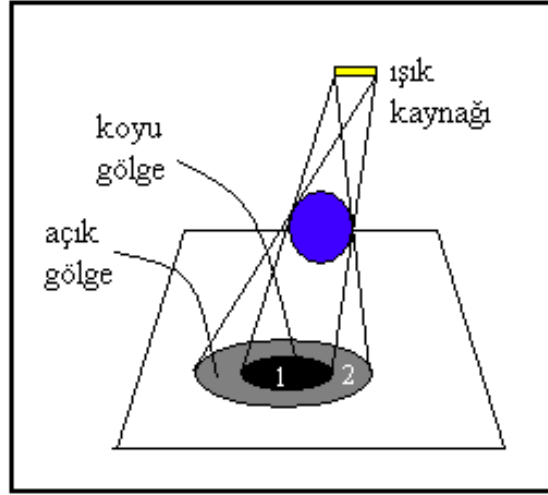
Şekil 2.3. Gölge modeli
