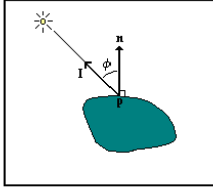
Şekil 1.21. Diffuse bileşen
