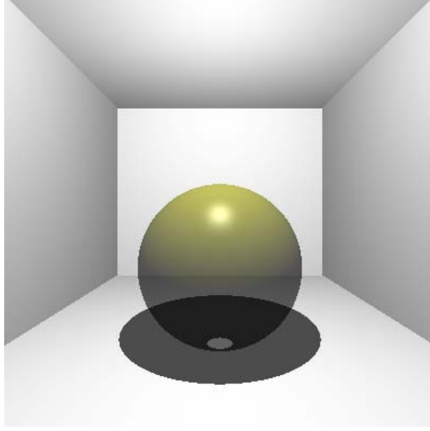
Şekil 2.9. Saydam küre
