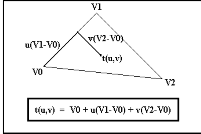
Şekil 1.5. Barisentrik koordinatlar
