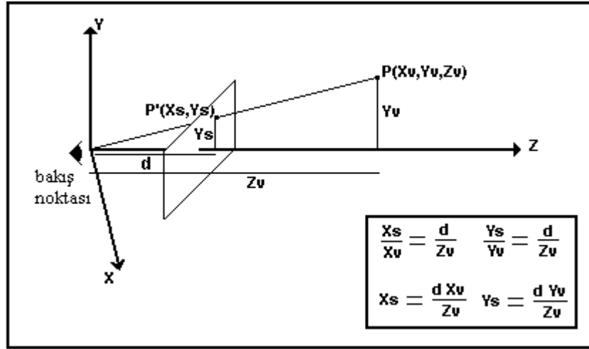
Şekil 1.7. Perspektif izdüşüm
