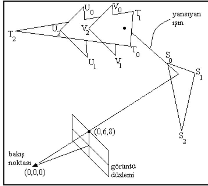
Şekil 1.18. Yansıma örneği
