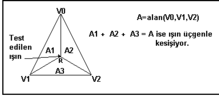
Şekil 1.11. Alan testi
