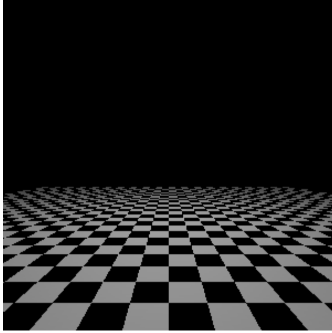
Şekil 1.29. Aliasing etkisi
