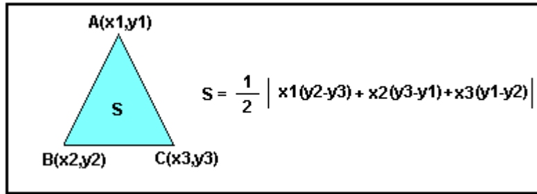
Şekil 1.12. Alan hesabı
