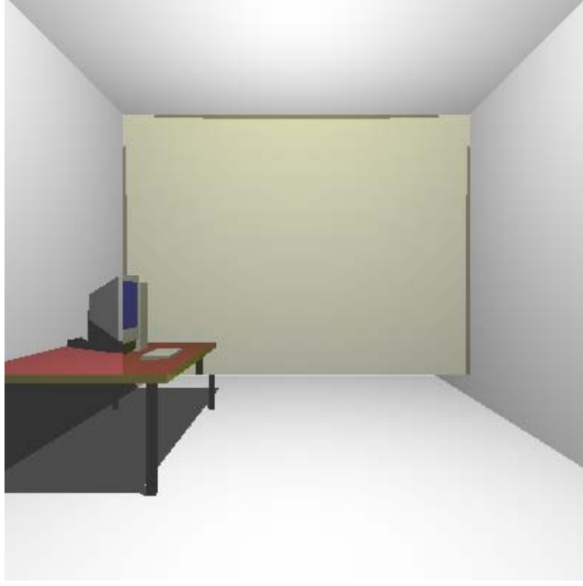
Şekil 2.10. Kırılma yüzey, n_1=1.0 , n_2=1.33
