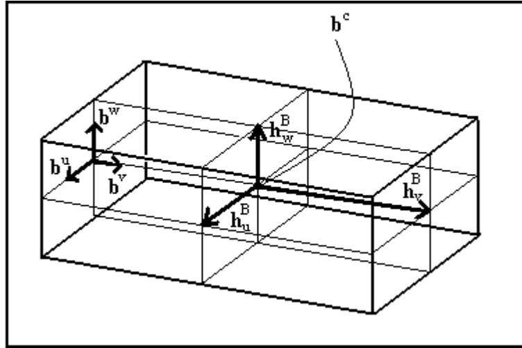
Şekil 1.34. Dikdörtgen prizma
