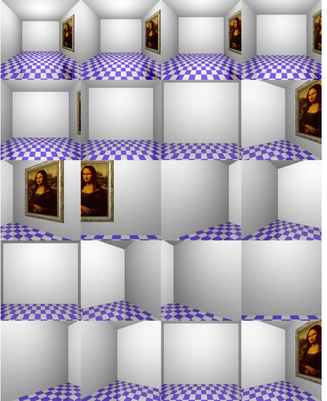
Şekil 2.23. Etkileşimli ışın izleme ile üretilen görüntüler
